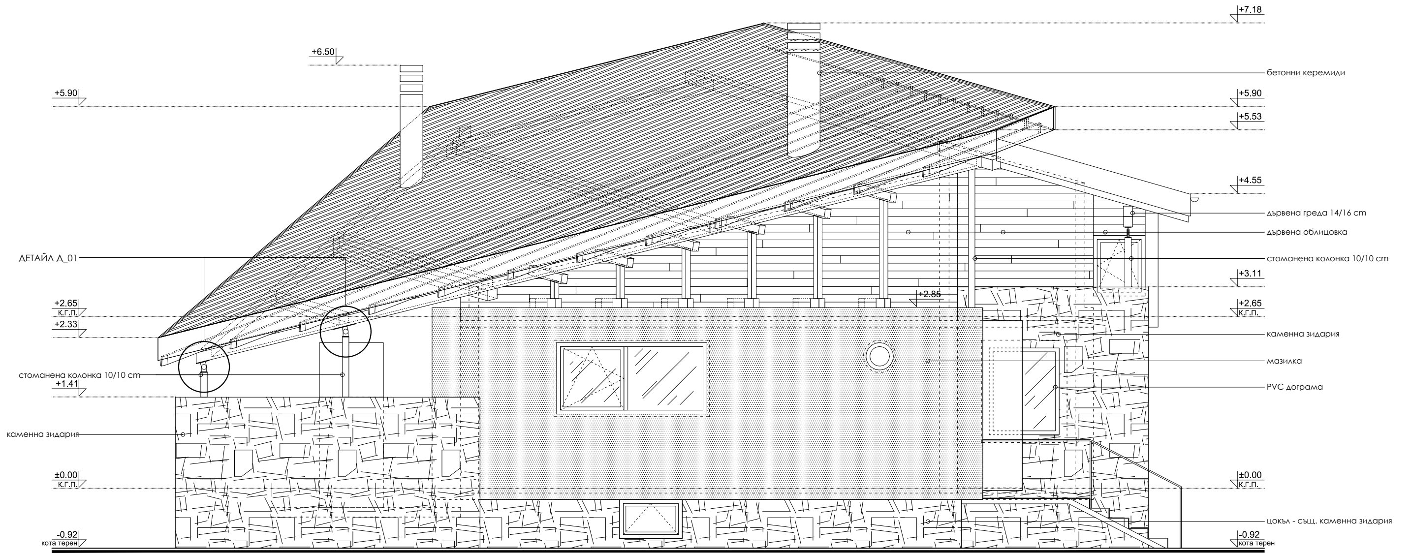
ФАСАДА ЮГОЗАПАД
