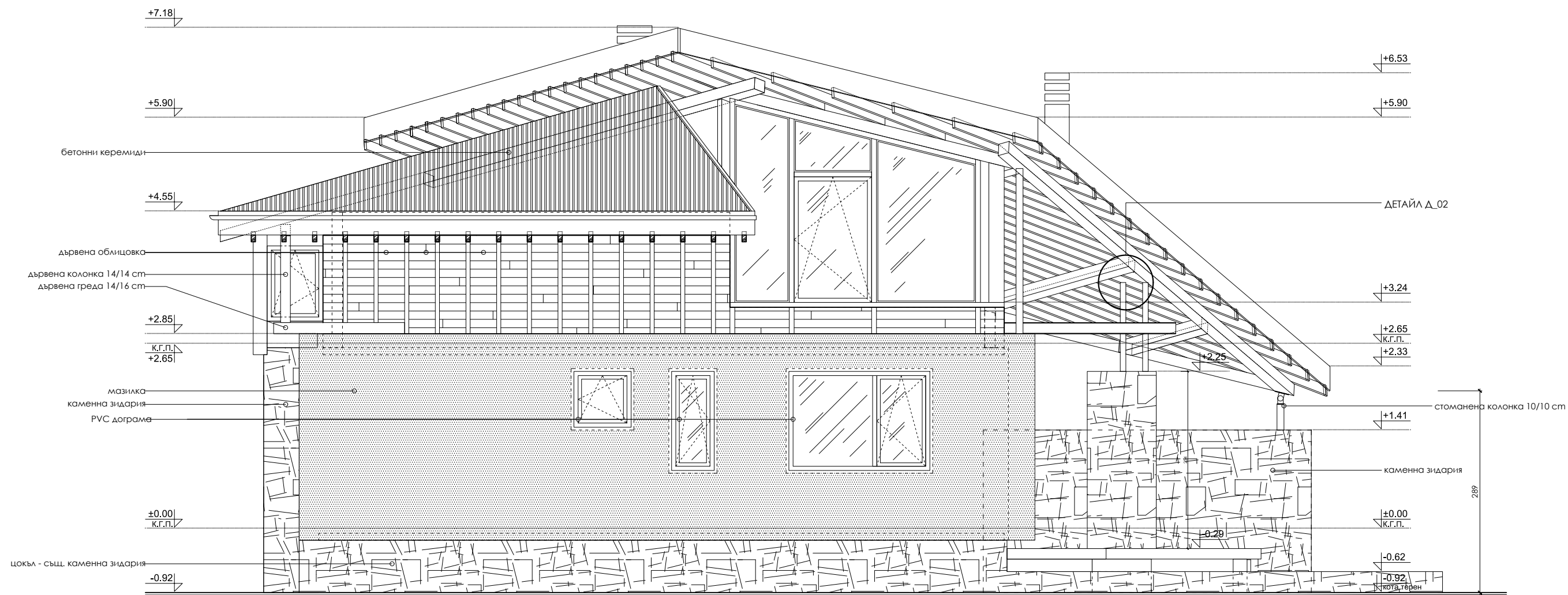
ФАСАДА СЕВЕРОИЗТОК
