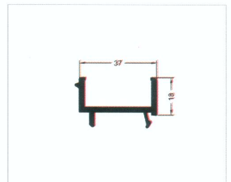
Държач за подвижен ламел
